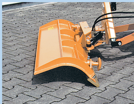
Federklappen-Räumschild mit Neigungswinkelverstellung
